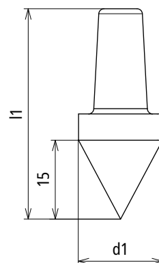
Maßbild SSP TE 20 TGTZN
