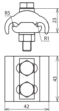
Maßbild PV 5.12.5 SKM8X45 GSG CUGALSN
