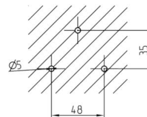
Bohrbild a)
