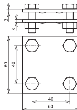
Maßbild KS FL30 STTZN
