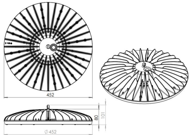
Abb. 2: Maße des SUN 245
