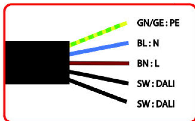
Abbildung 6 – Anschlussdiagramm
