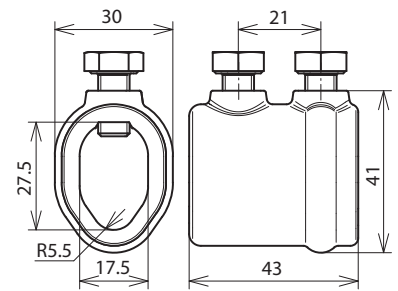
Maßbild TM G 7.10 16 ZG
