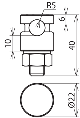
Maßbild KSV 6.10 FER V2A
