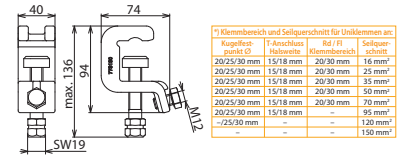
Maßbild UK 30 SK
