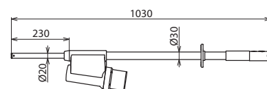
Maßbild PHE4 6.6 S
