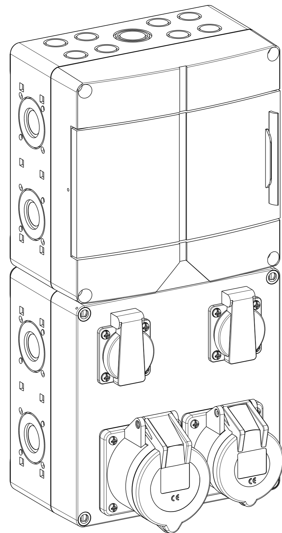
STV 922-S STV 922-K
