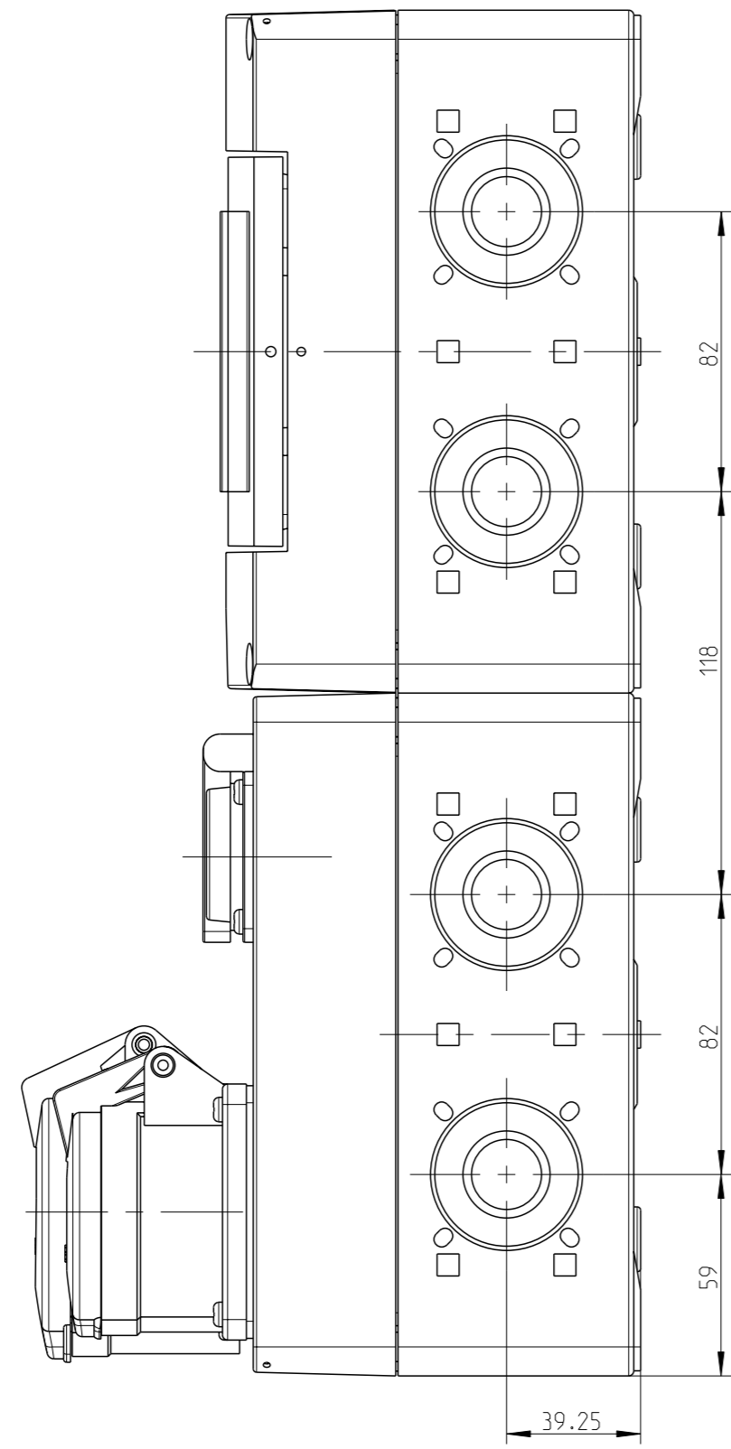
STV 922-S STV 922-K
