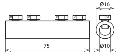
Maßbild VM 8 SKM6X8 AL
