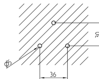
Bohrbild
