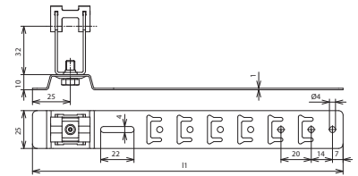
Maßbild DLH UG 8 H32 L475 V2A
