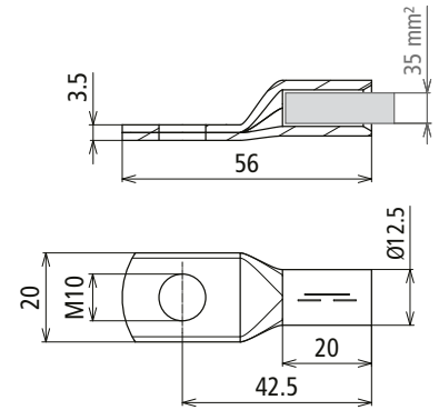
Maßbild PKS 35 10 CUGALNISN
