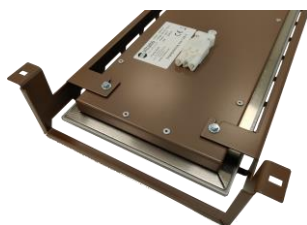
Einspeisung mittels mitgeliefertem Buchsendeil
