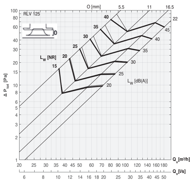
Druck-Volumenstromkennlinie Zuluft
