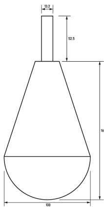
Maßzeichnung Gruppenansicht
