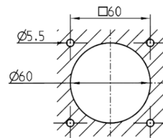
Montageausschnitt
