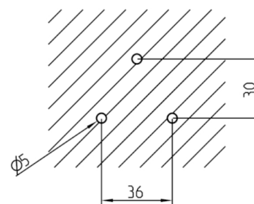
Bohrbild
