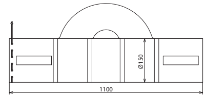
Maßbild STT 110 15
