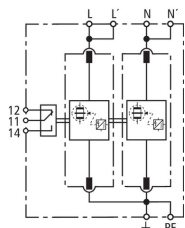
Prinzip Schaltbild DV M TN 255 FM
