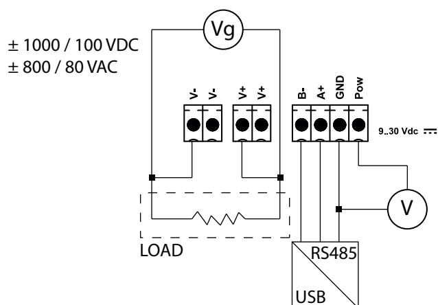
Anschlussschema BT7300 / BT7350
