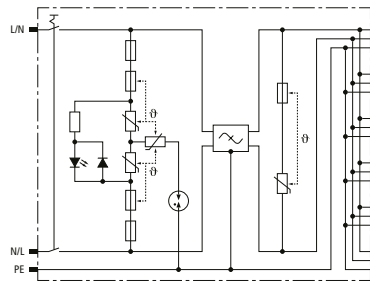
Prinzipschaltbild
