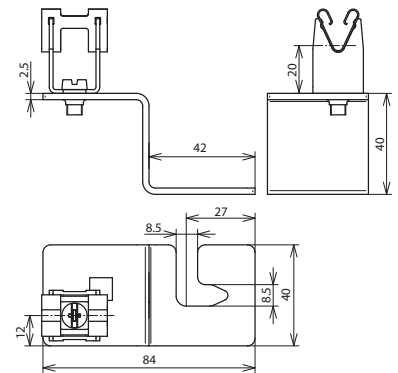
Maßbild DLH DG 8 TD B8.5 V2A
