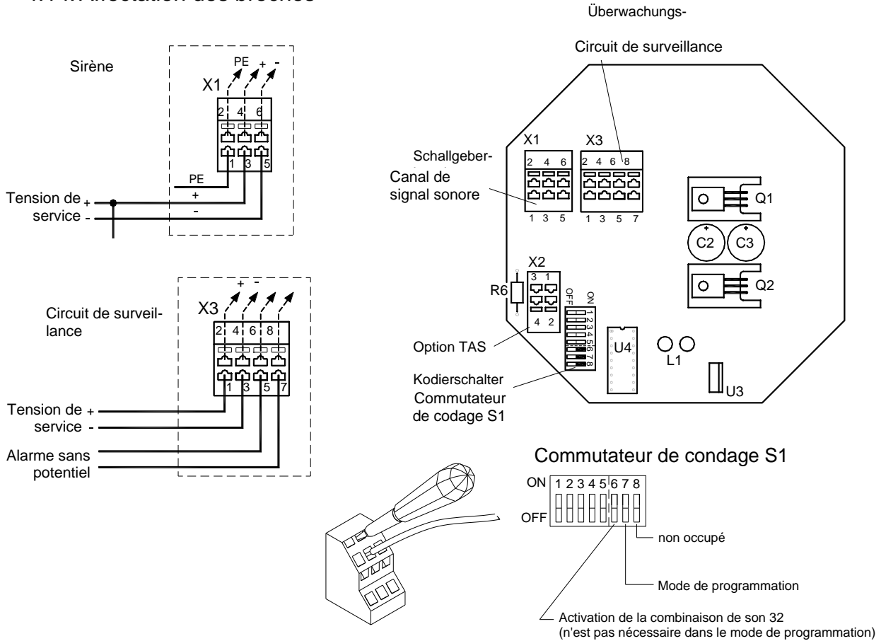
Fig. 10 Affectation des broches et éléments de commande
