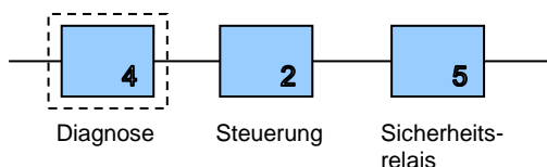
Abb. 6 Sicherheitsrelevantes Blockdiagramm
