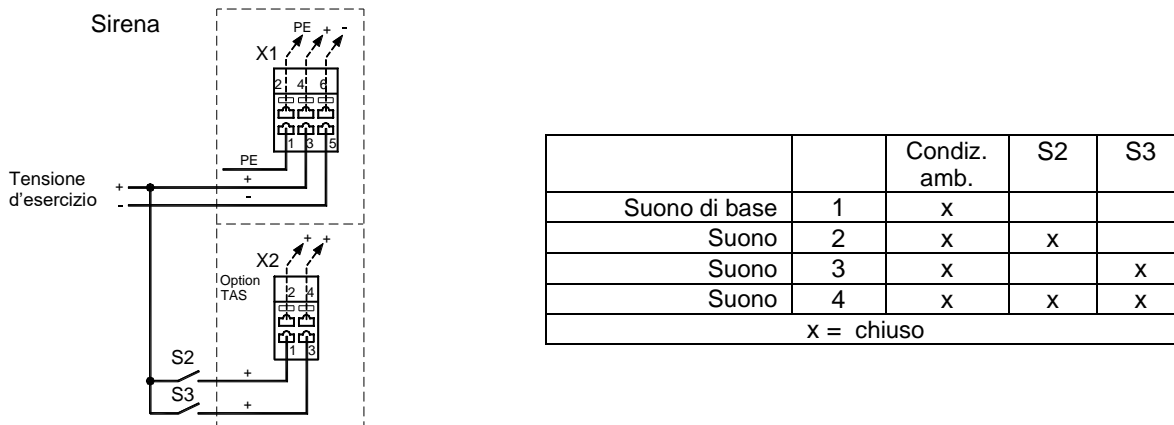
Fig. 11 Assegnazione delle connessioni, opzione TAS
