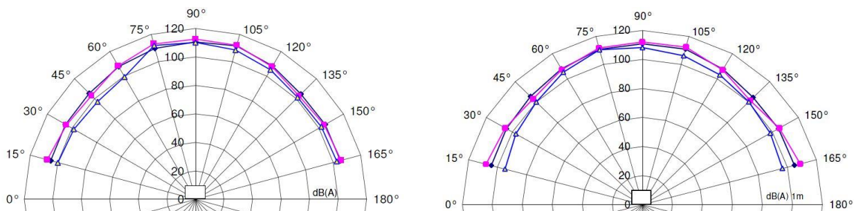
DS 10 Intensità sonora, diagramma orizzontale
