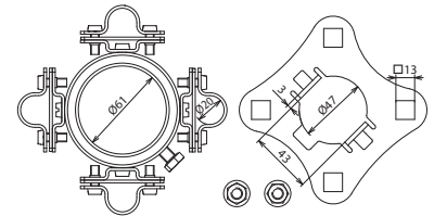
Maßbild BFS D61 4X20
