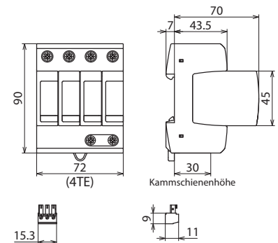
Maßbild DG M TNS ACI 275 FM
