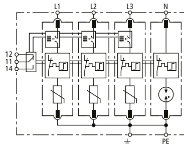
Prinzip Schaltbild DG M TNS ACI 275 FM
