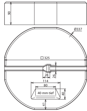
Maßbild
