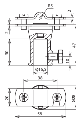
Maßbild
