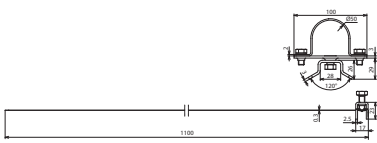
Maßbild
