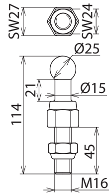
Maßbild KFP 25 M16 45 SSM
