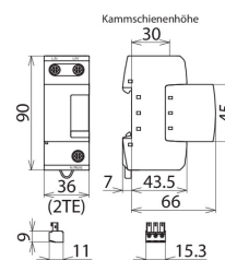
Maßbild DB M 1 150 FM
