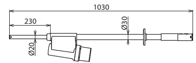
Maßbild PHE4 6 S
