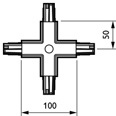
3-circuit square ZCS750
