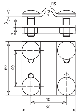
Maßbild KS 8.10 FL30 FRSM8 STTZN
