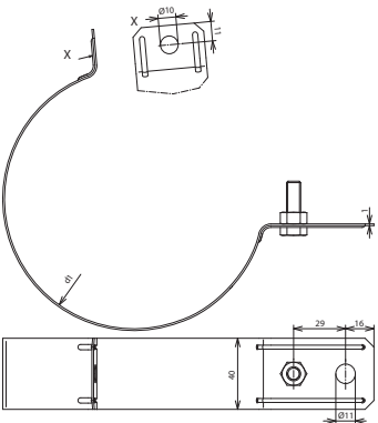
Maßbild RRS 100 B11 STTZN
