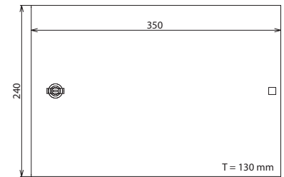
Maßbild DPG LSA 60 P
