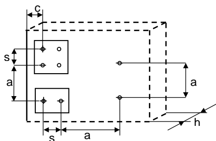
Anordnung der Rand- und Achsabstände in Beton, Verankerungsgrund Gruppe „a“
