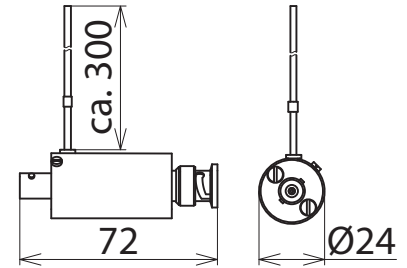
Maßbild UGKF BNC
