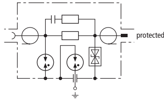
Prinzipschaltbild UGKF BNC
