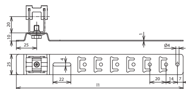
Maßbild DLH UG 8 H20 L205 CU
