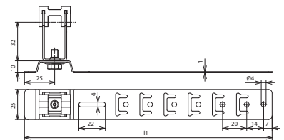
Maßbild DLH UG 8 H32 L335 V2A
