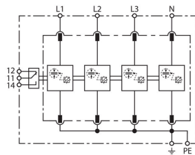
Prinzipialschaltbild DV M2 TNS 255 FM
