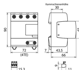
Maßbild DVA EMOB M 3P 255 FM
