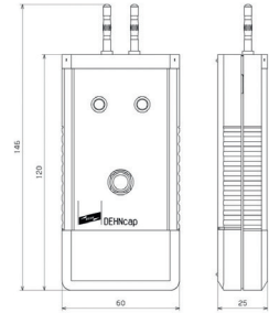
Maßbild SPG DCA IT LRM
