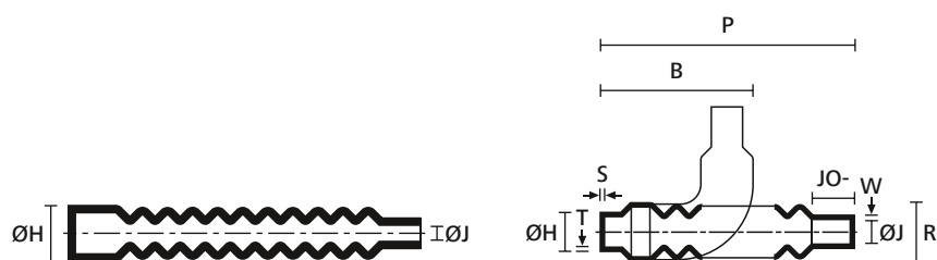
a: Ungeschumpftes Formteil (Lieferzustand)
