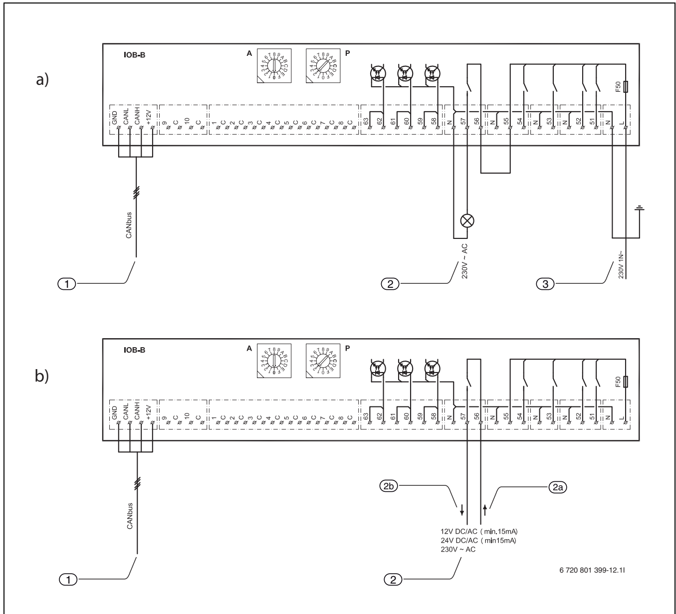
Joon. 25 Ühenduskeem. a) 230 V väljundsignaal b) potentsiaalivaba kontakt
