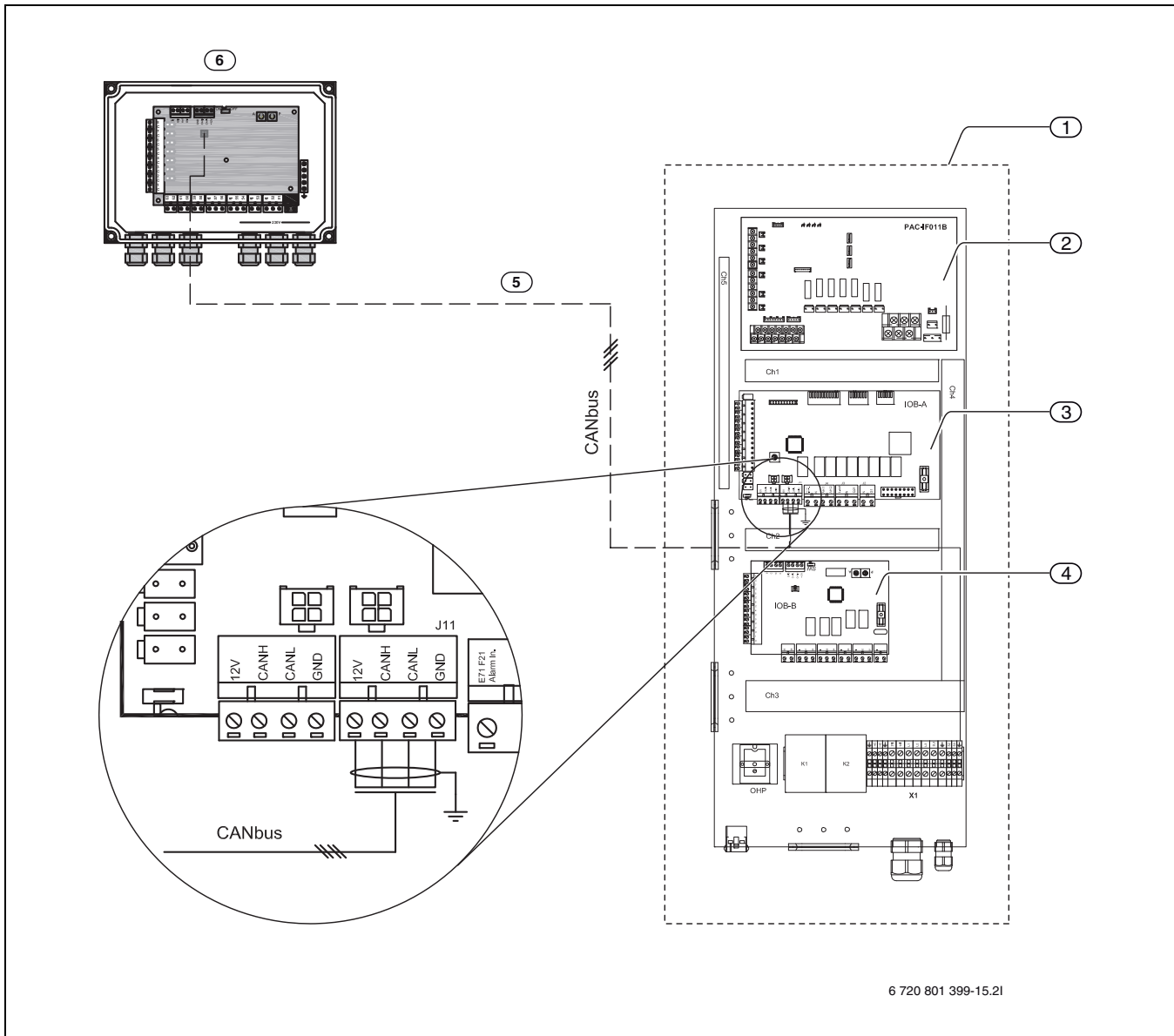
Afb. 17 Aansluiting op de hoofdprintplaat in de binneneenheid van de warmtepomp
