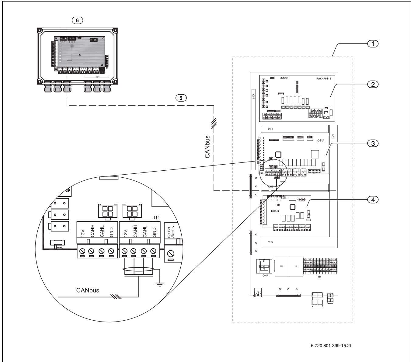
Рис. 71 Подключение к главной плате во внутреннем блоке теплового насоса
