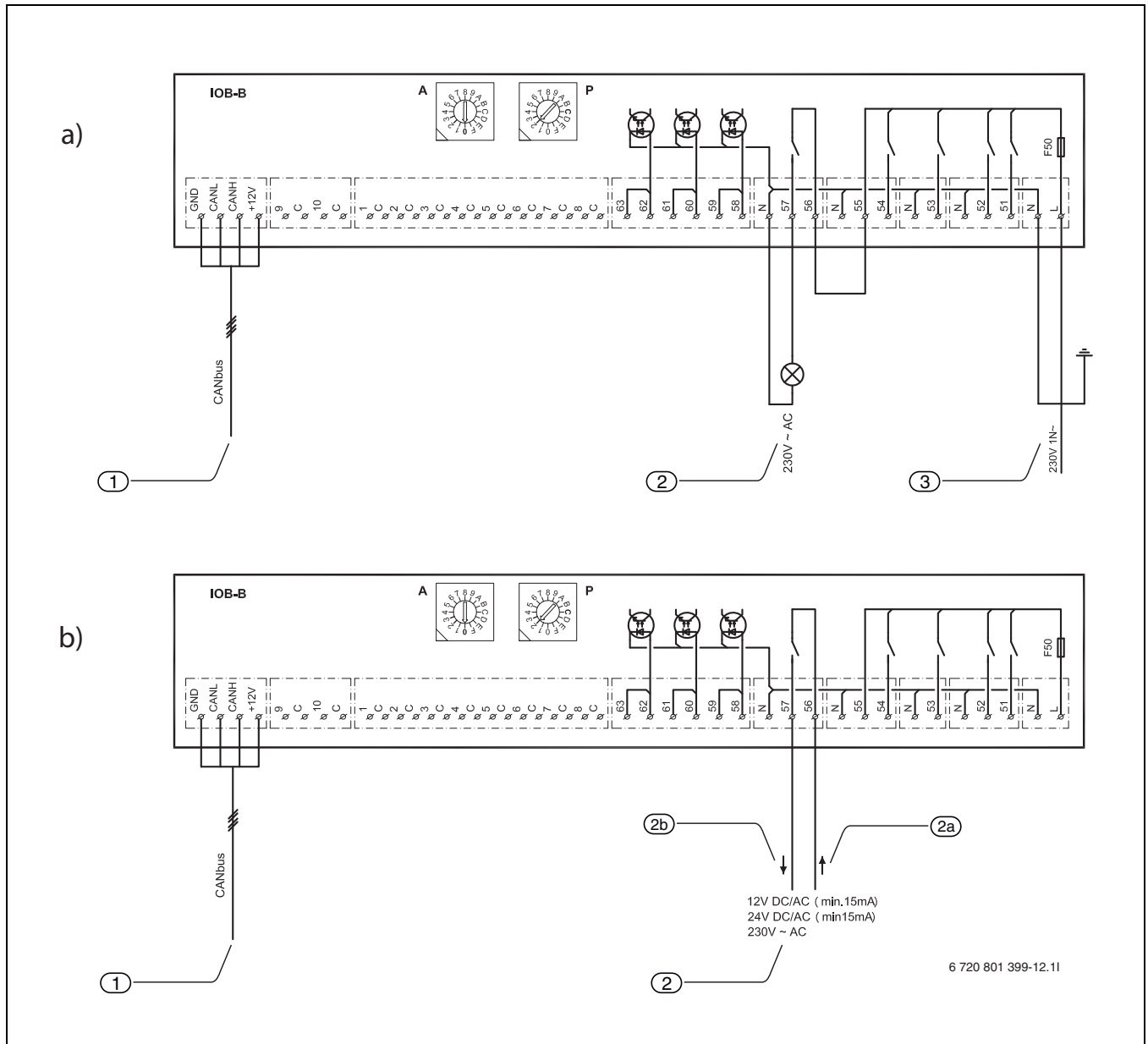
Bild 34 Schaltplan. a) 230 V Ausgangsignal b) Potentialfreier Kontakt
