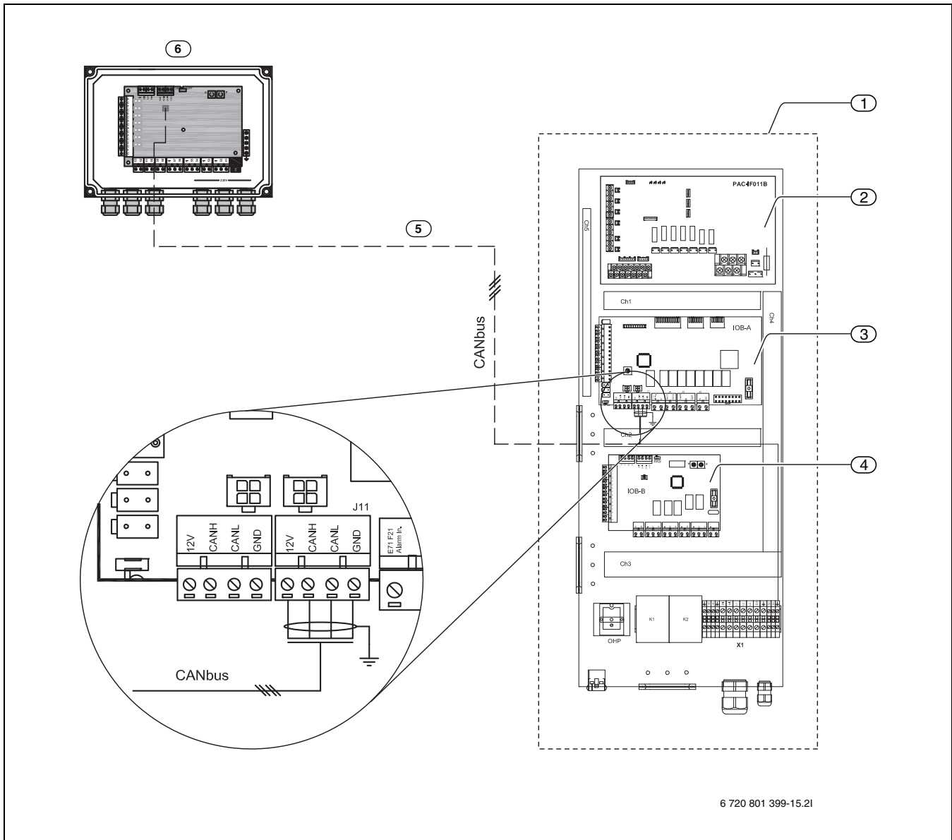
Pav. 53 Prijungimas prie pagrindinės plokštės šilumos siurblio vidiniame bloke
