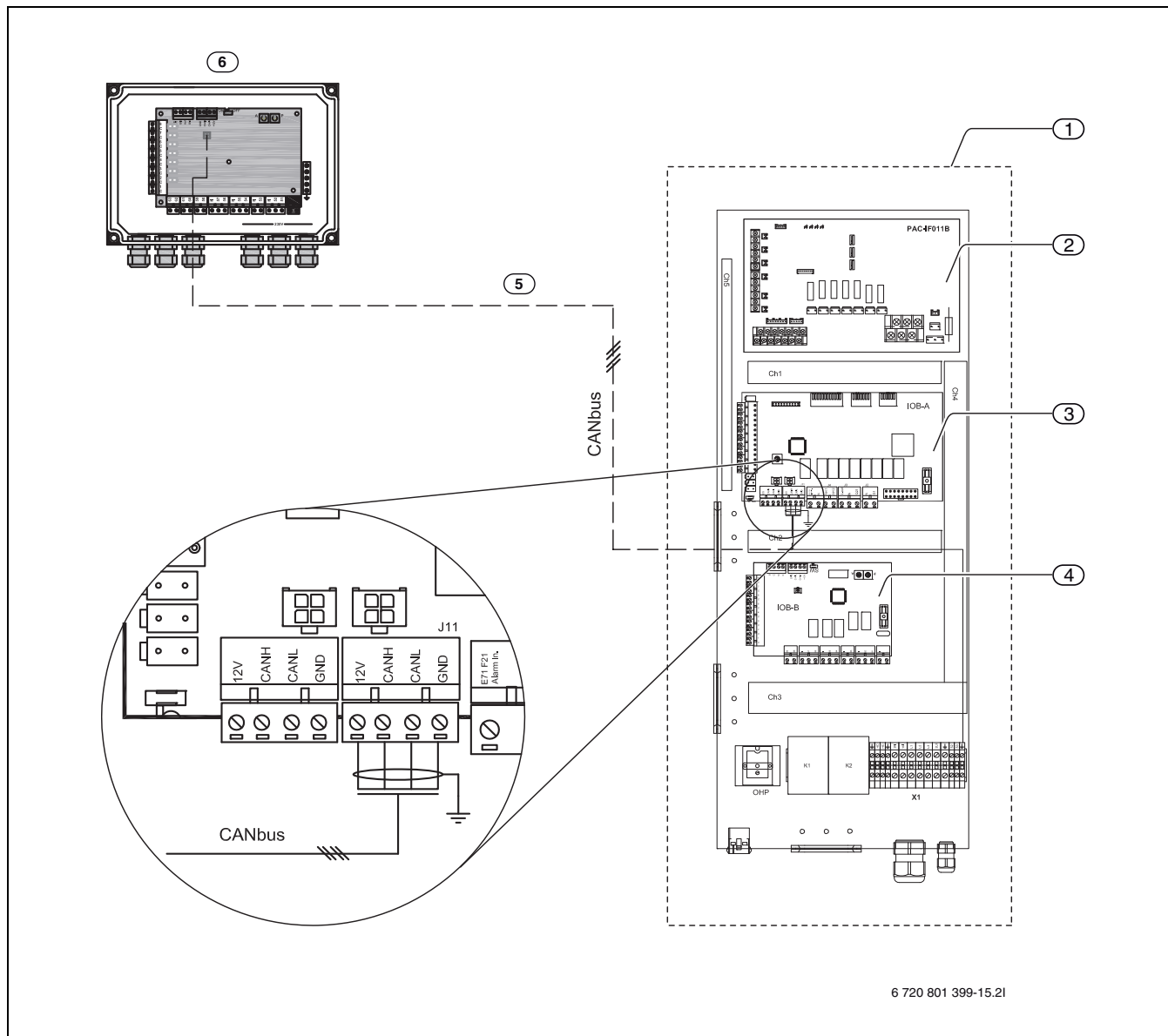
Sl. 62 Priklučitev na glavno vezje v notranji enoti toplotne črpalke
