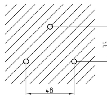
Bohrbild
