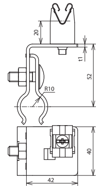
Maßbild DLH DG 8 RSF20.25 V2A
