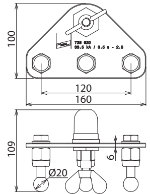
Maßbild EAPA 3 KFP 20 KKH
