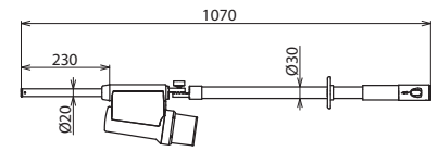
Maßbild PHE4 6 S ZK
